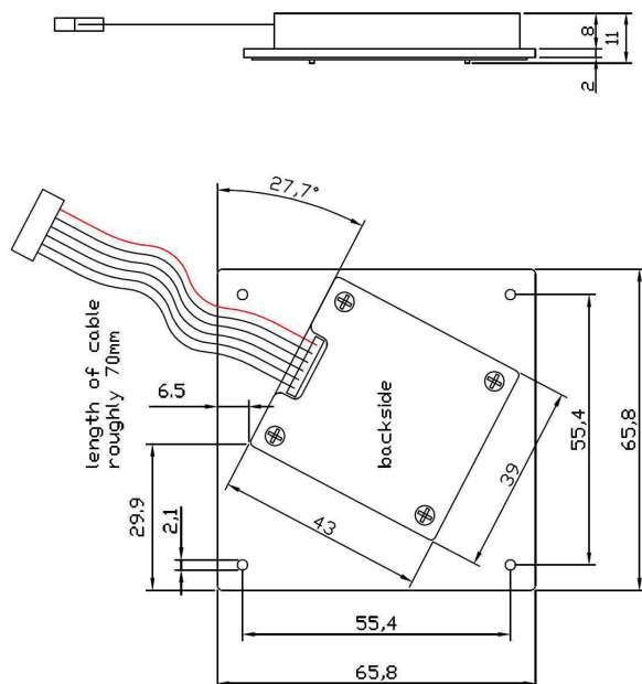
图 10 IVS-148 模块尺寸 (单位: mm)
