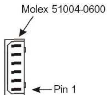
图 5 IVS-148 接口示意图
