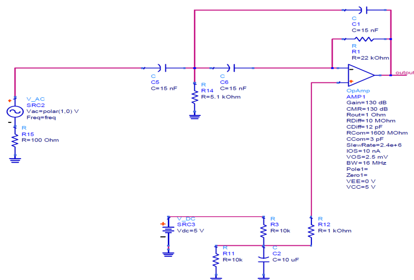
图 8 增益为 0dB、频率为 1kHz 的高通滤波放大电路
