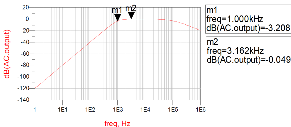
图 9 频率响应
