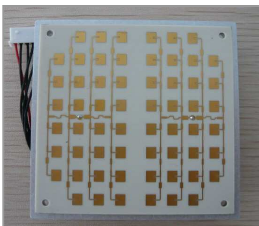
图 1 IVS-148 天线面实物图
