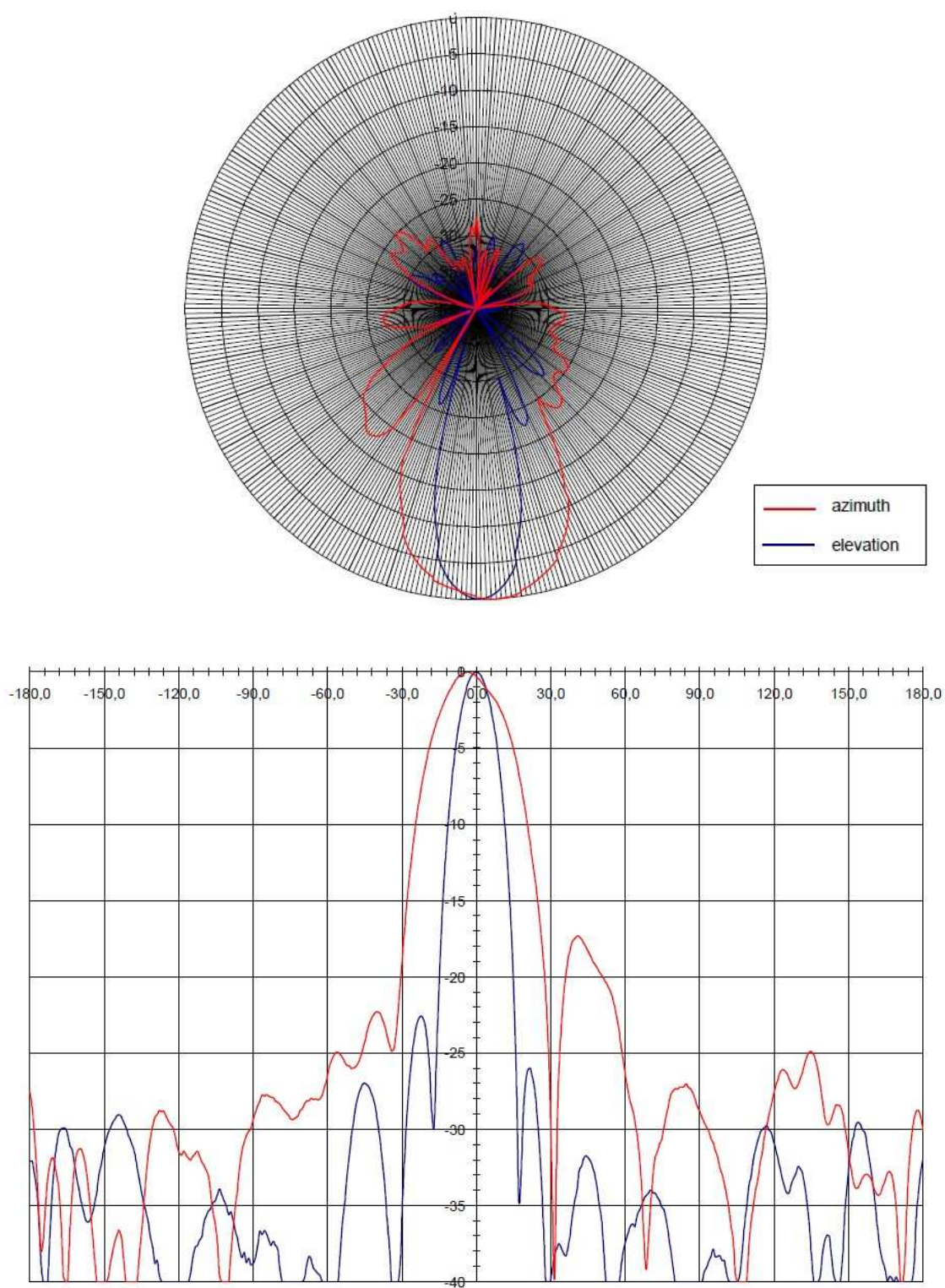
图 4 天线辐射方向图
