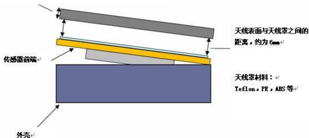
图 12 雷达传感器天线罩安装示意图
